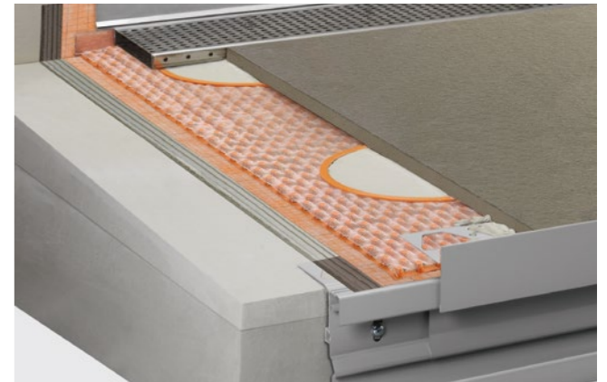
Losse plaatsing op Schlüter-KERDI en Schlüter-TROBA-PLUS 8G
