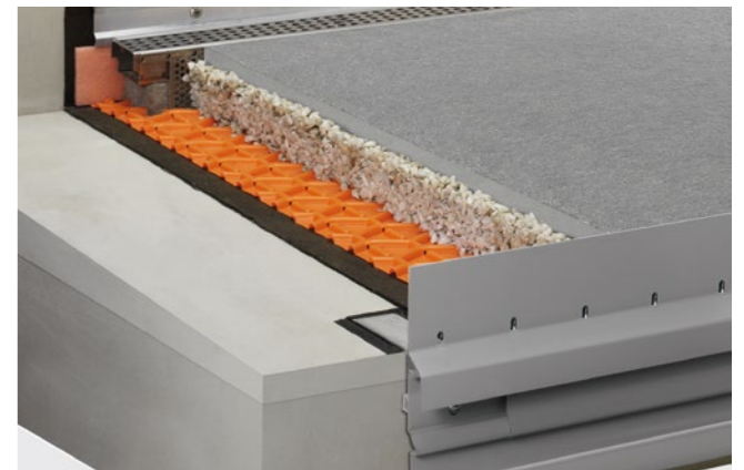
Bekledingsconstructie op kiezel-/splitbed met Schlüter-TROBA
